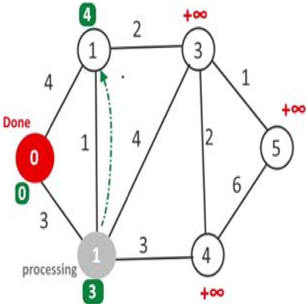
Dijkstra Algorithm
